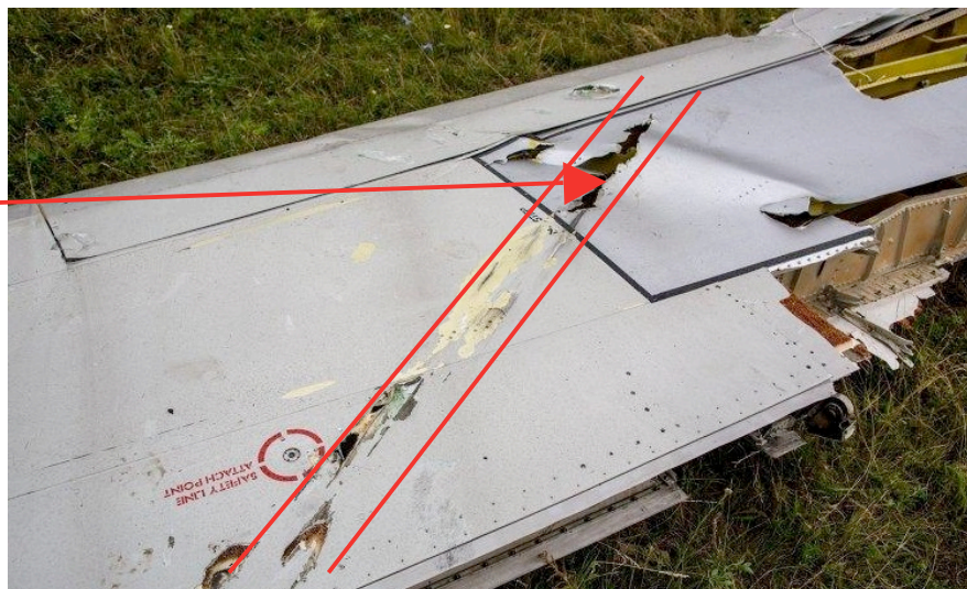
Фото 19. Повреждения плоскости Boeing 777
